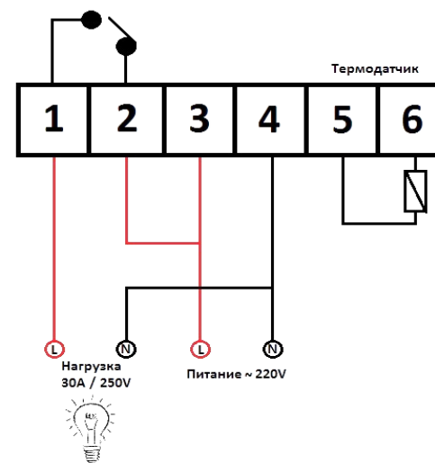
Схема подключения терморегулятора Ringder RC-114M30A
